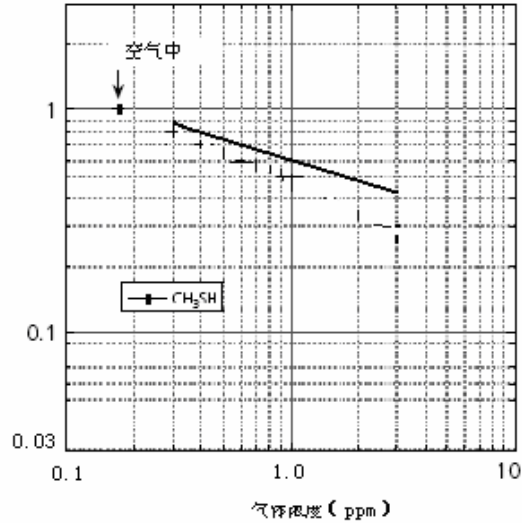
图3 灵敏度特性
