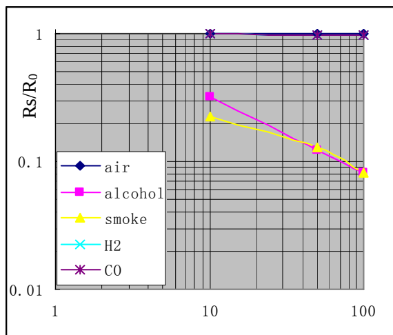
图3： 传感器典型的灵敏度特性曲线
