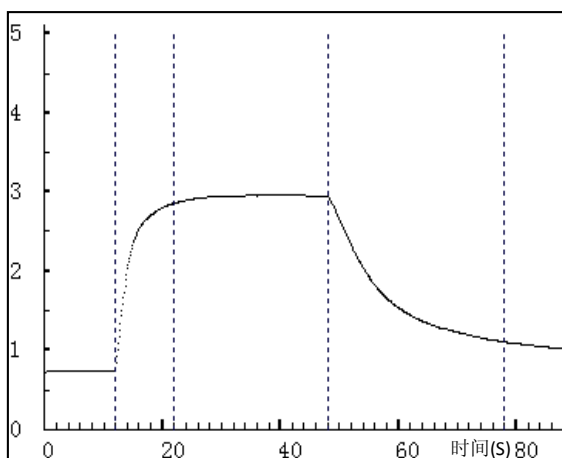
图5： 响应恢复曲线
