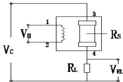
图2： MP135A 测试电路
