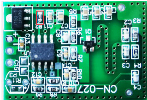
R2 增大感应输出时间变长
