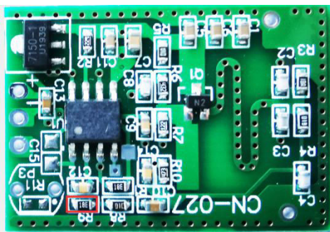
R9 增大感应距离变长，反之变短
